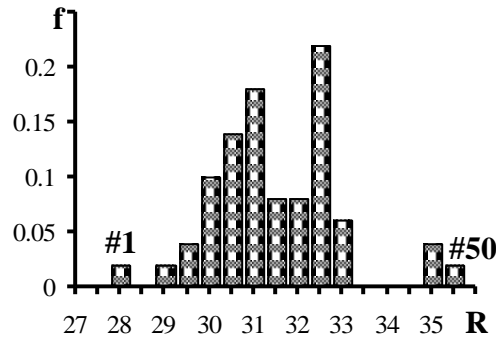
Рис. 1. Гістограма міцності композиту
